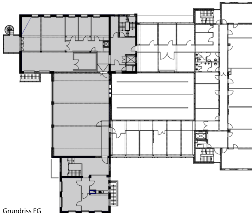
Grundriss EG
